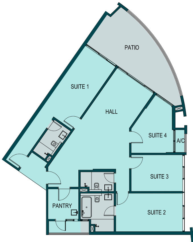
TYPE J 3+1BR-A
