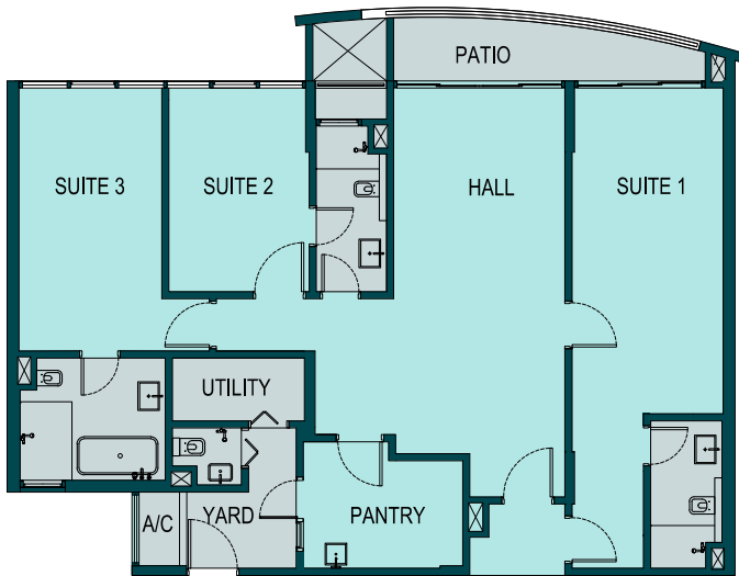
TYPE I 3BR-C
